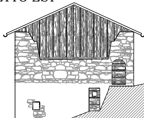
PROSPETTO EST
