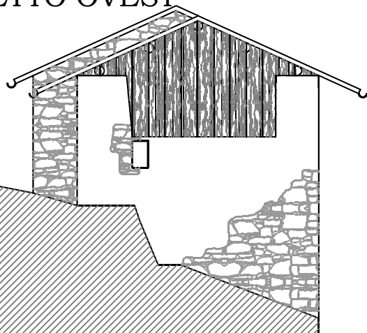
PROSPETTO OVEST
