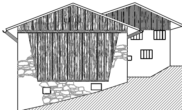
PROSPETTO OVEST
